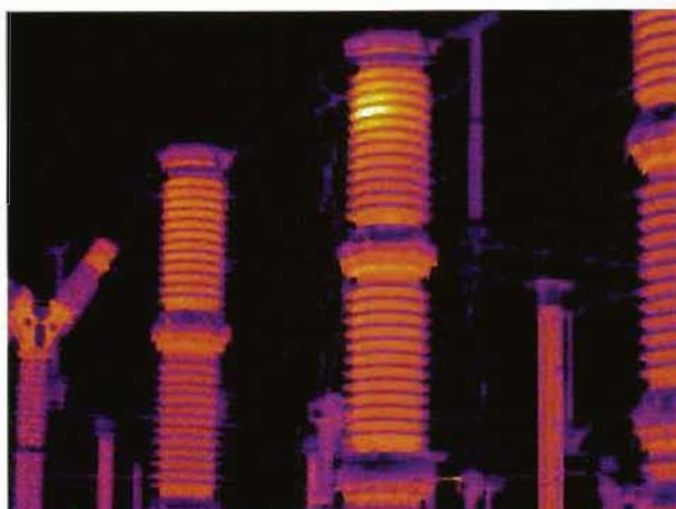
图 J. 20 220kV 避雷器发热
