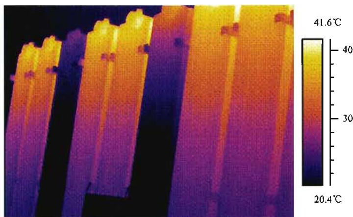
图 J.1 变压器散热器进油管关上
