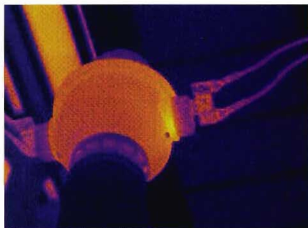
图 J. 9 互感器内接头发热
