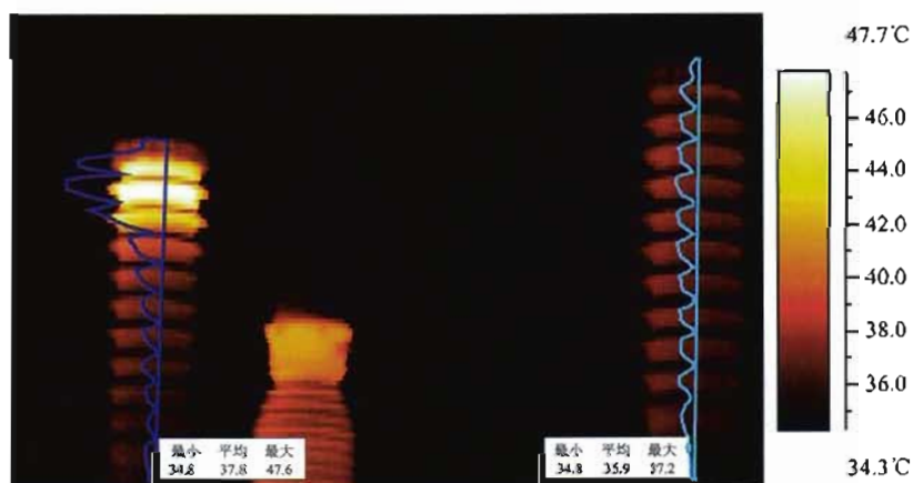
图 J. 10 耦合电容器电容量减少 10%，引起发热
