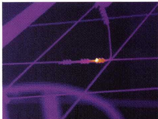
图 J. 44 线路夹头发热，接触不良
