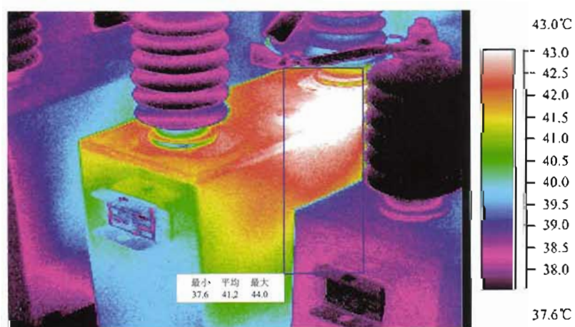
图 J. 14 电容器局部发热
