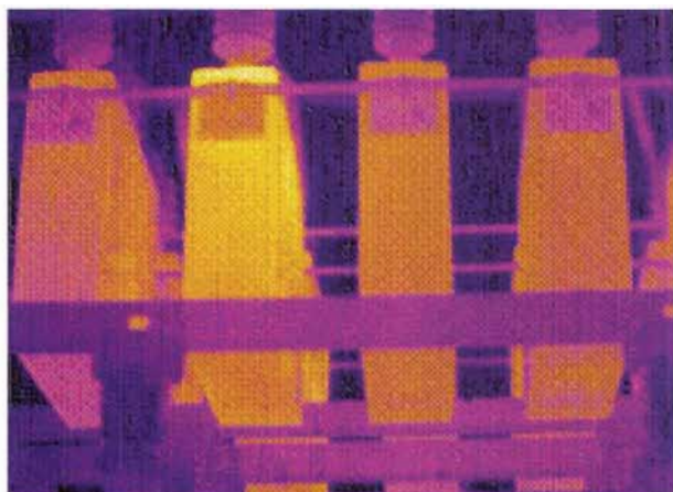
图 J. 15 电容器介质损耗偏大引起发热
