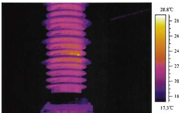
图 J. 34 套管伞裙套粘接不良发热
