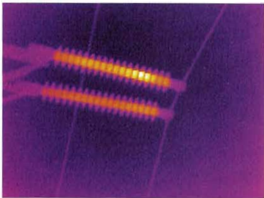
图 J. 37 合成绝缘子内部受潮，发热
