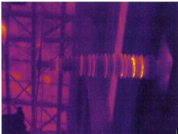
图 J. 32 穿墙套管发热，套管外表污秽
