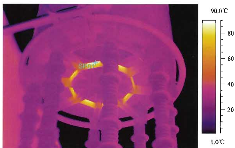
图 J. 50 平波电抗器低负荷涡流发热
