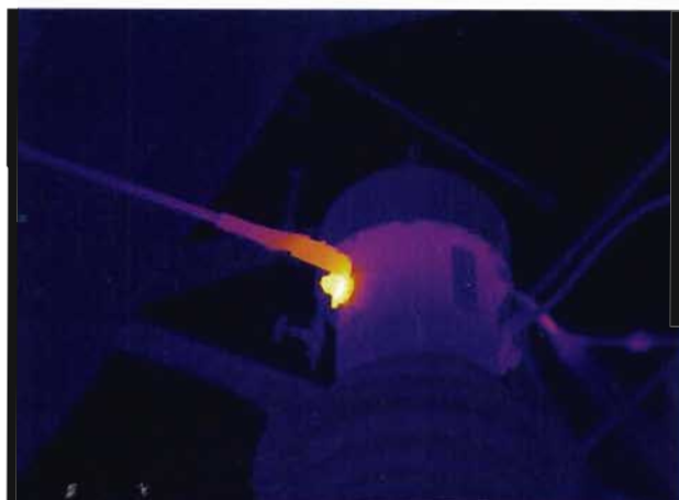
图 J. 8 电流互感器接头发热
