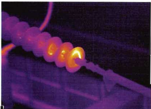
图 J. 39 瓷绝缘子发热，表面污秽
