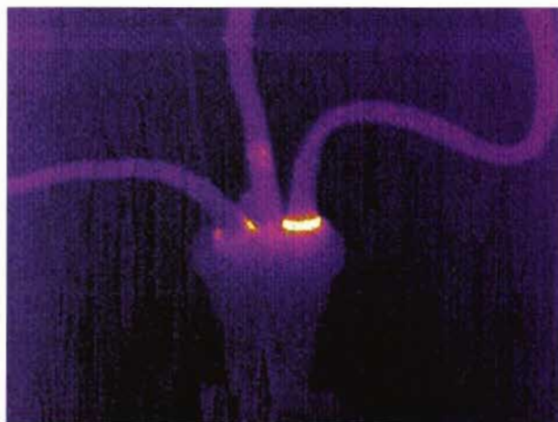
图 J.24 10kV 油纸电缆接头发热， 分相处电容放电
