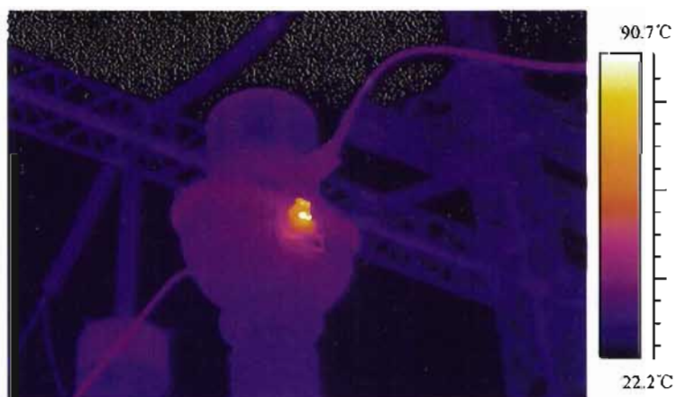
图 J.7 互感器变比接头发热
