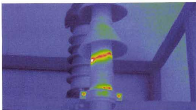
图 J. 27 电缆护套受损，发热
