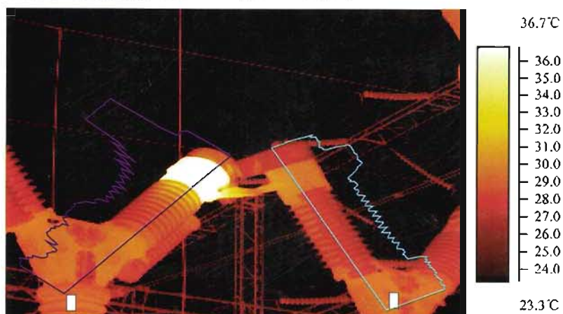
图 J.46 断路器内静触头发热，接触不良
