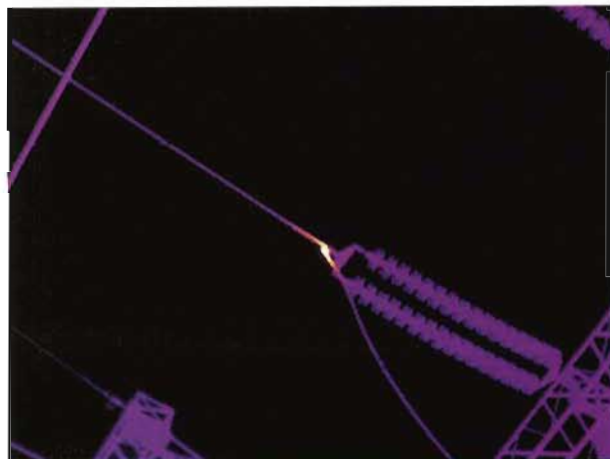
图 J. 42 220kV 线夹发热，接触不良
