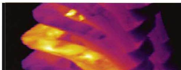
图 J. 52 水轮机接头不良，发热
