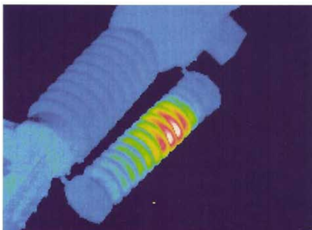
图 J. 17 断路器并联电容发热
