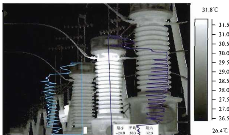
图 J.6 互感器介质损耗偏高发热，B 相
