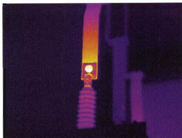
图 J. 29 35kV 电缆接头发热，接触不良
