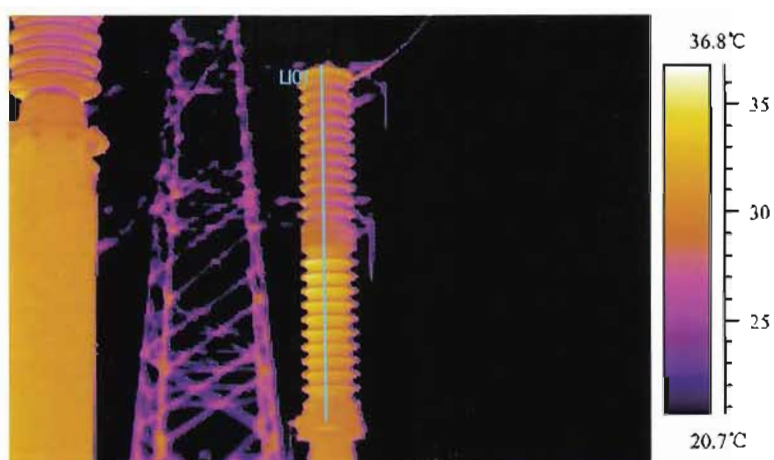
图 J. 12 耦合电容器下节介质损耗偏大发热
