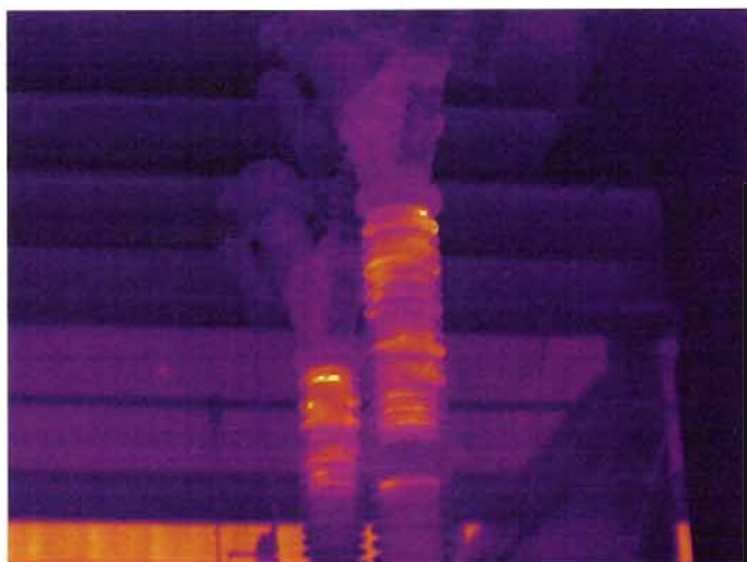
图 J. 49 断路器支柱发热，支柱瓷套污秽
