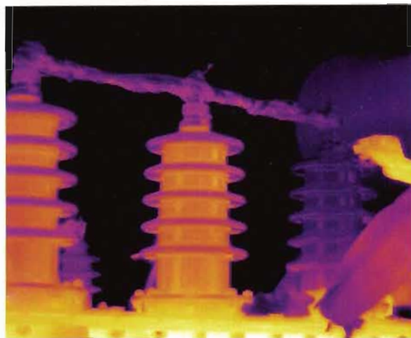
图 J. 36 变压器套管发暗，套管缺油
