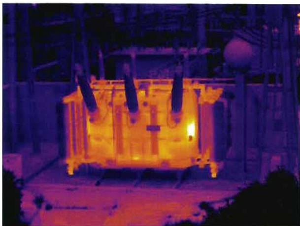
图 J.2 变压器磁屏蔽不良
