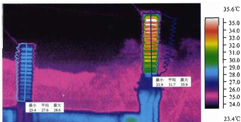
图 J. 11 耦合电容器介质损耗超标，发热
