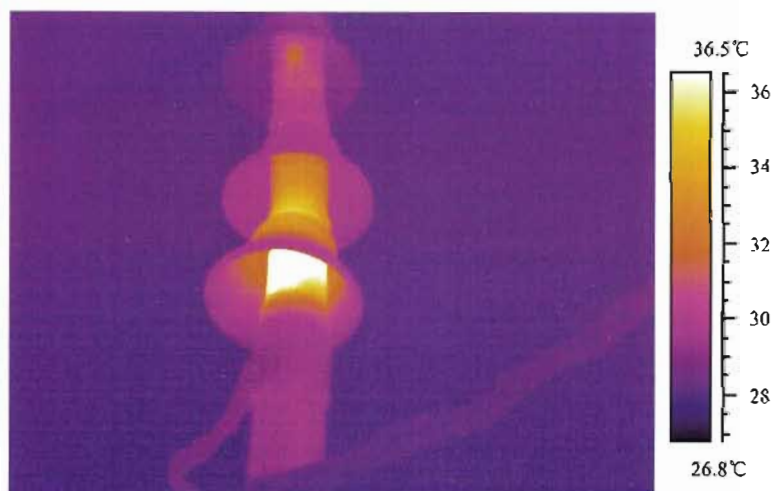
图 J.25 电缆头包接不良，发热
