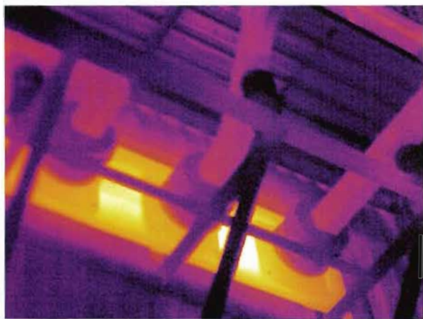
图 J. 35 穿墙套管的钢板发热，电磁环流
