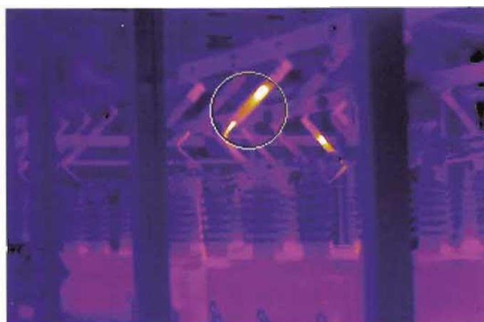
图 J. 13 电容器熔丝发热
