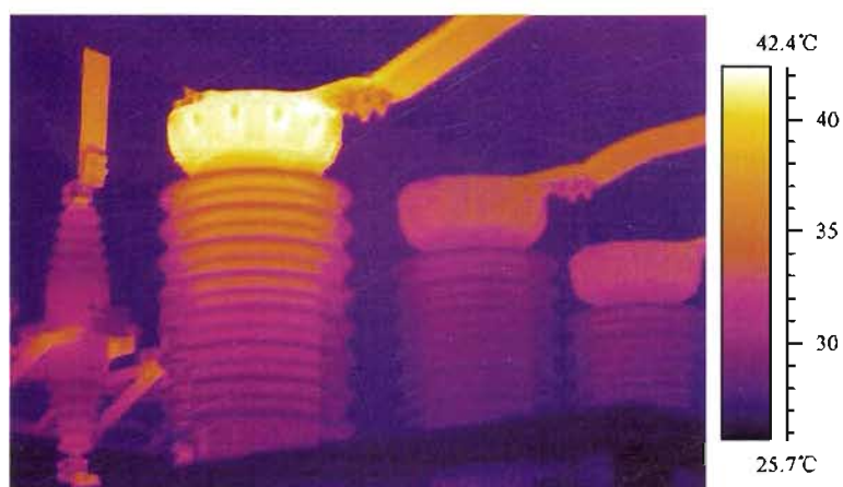
图 J.48 断路器触头发热，内部接触不良
