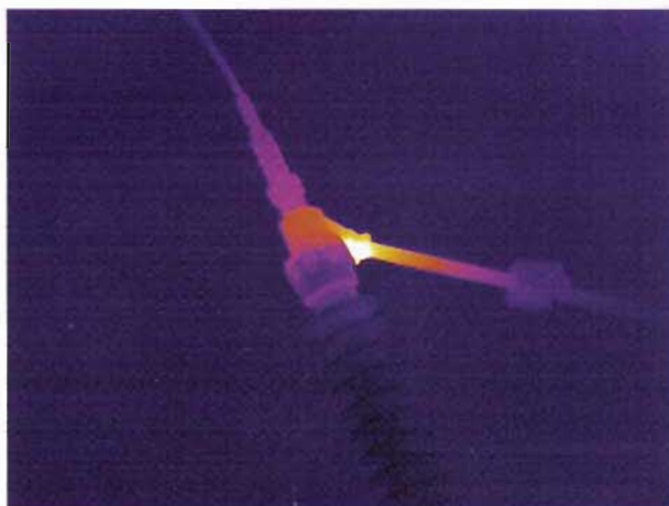
图 J. 43 隔离开关内转头发热，接触不良
