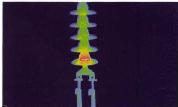
图 J. 40 瓷绝缘子低值，发热
