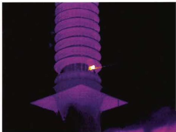
图 J. 16 耦合电容器电容接头发热
