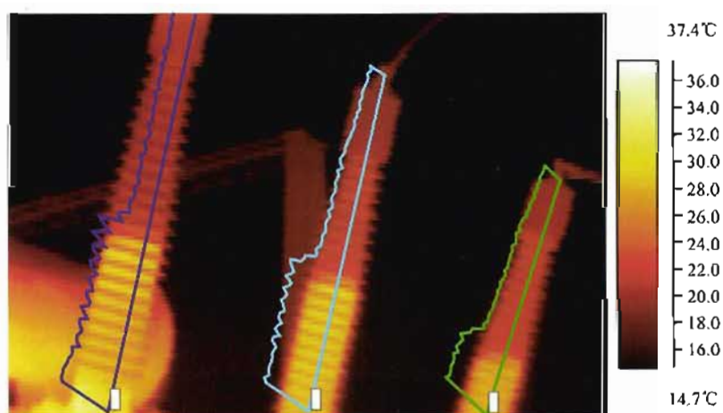
图 J. 30 变压器的套管温度异常，套管缺油
