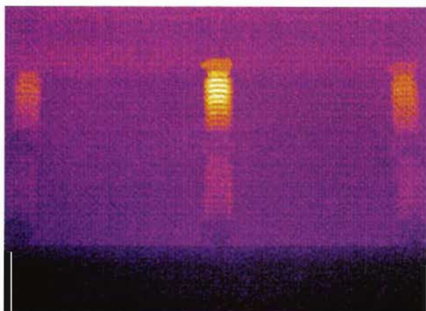
图 J. 18 220kV 氧化锌避雷器发热
